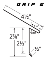
DRIP EDGE
